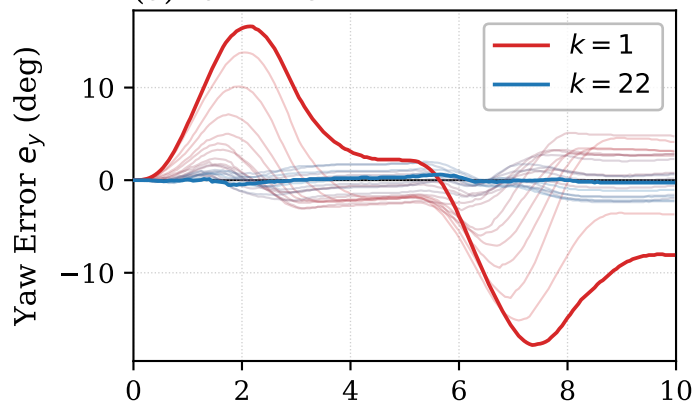
(d) Yaw Error
